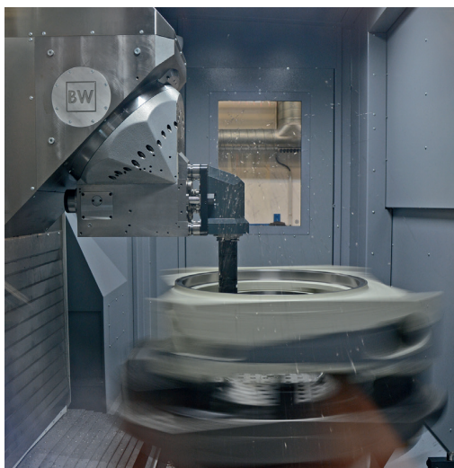
2 Geklemmter Schwenkopf mit Drehwerkzeughalter und schnell drehender Torquetisch in Aktion; die Unwuchtkontrolle ist im Standard an Bord (Bild: Hanser)
